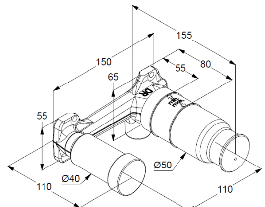
Maßzeichnung
