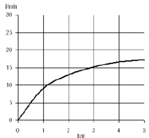
Durchflussdiagramm
